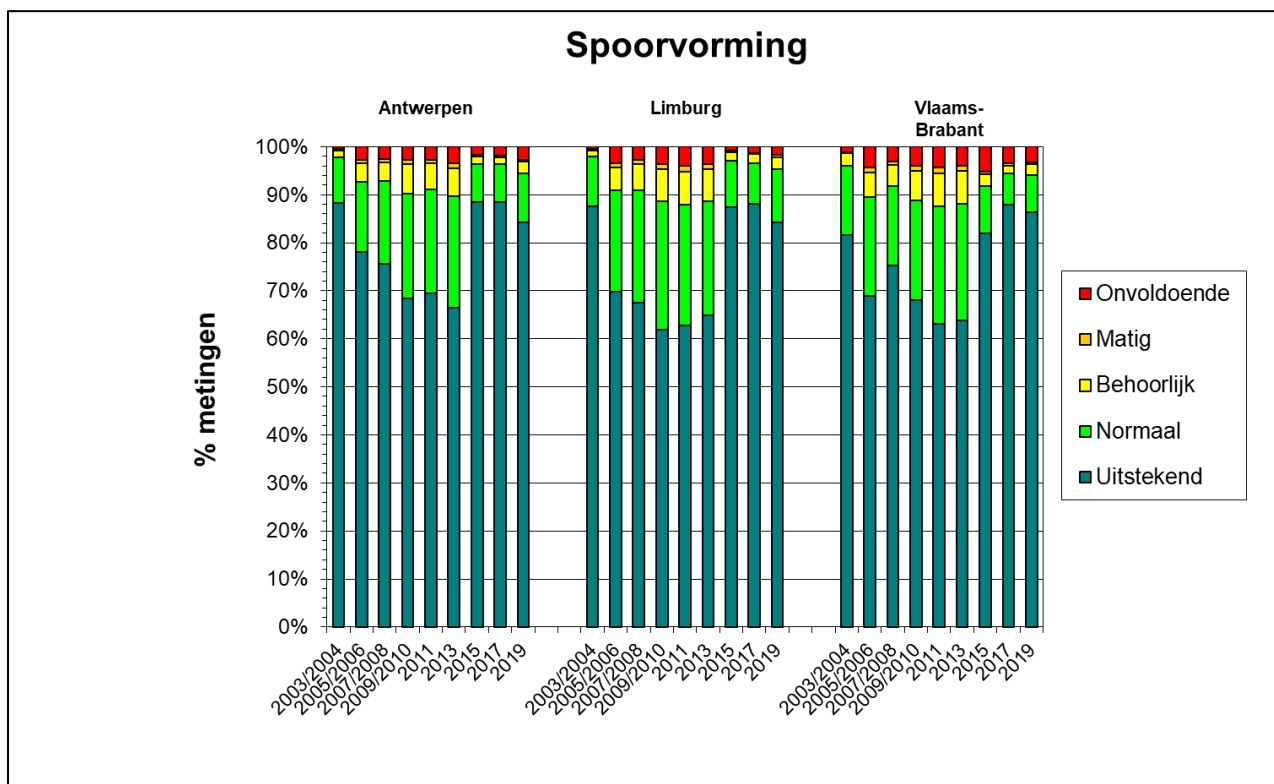
Figuur 2.1 Overzicht van de spoorvorming sinds 2003 voor Antwerpen, Limburg en Vlaams-Brabant
