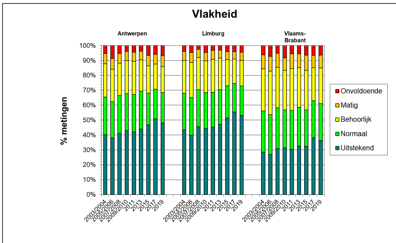
Figuur 2.5 Overzicht van de vlakheid sinds 2003 voor Antwerpen, Limburg en Vlaams-Brabant
