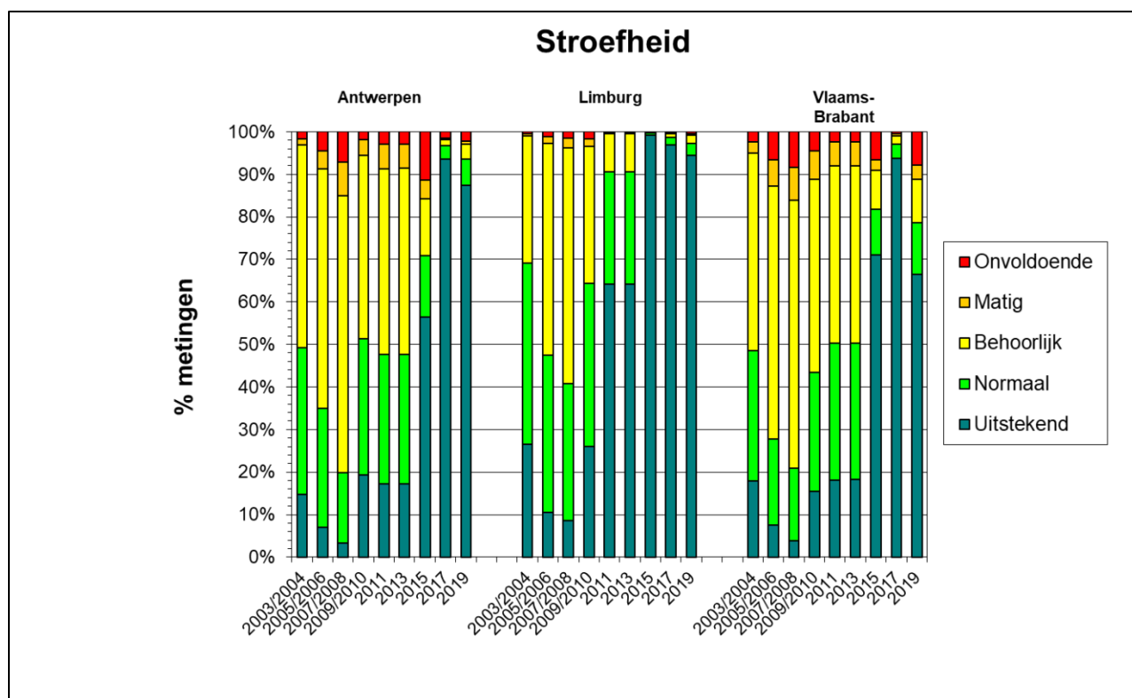
Figuur 2.2 Overzicht van de stroefheid sinds 2003 voor Antwerpen, Limburg en Vlaams-Brabant
