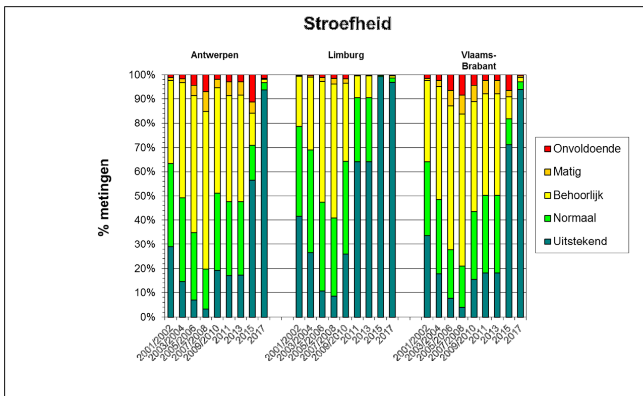
Figuur 2.2 Overzicht van de stroefheid sinds 2001 voor Antwerpen, Limburg en Vlaams-Brabant
